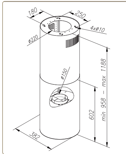
TUBUS W
