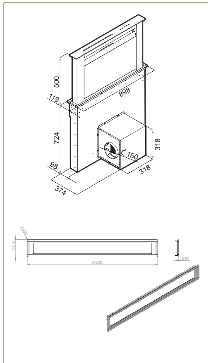
MOONDRAFT / 90 CM
