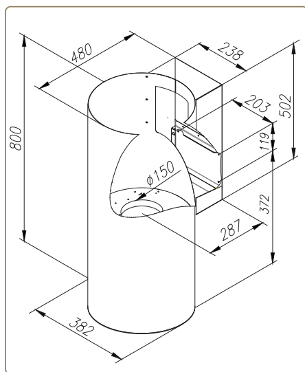
TUBUS
