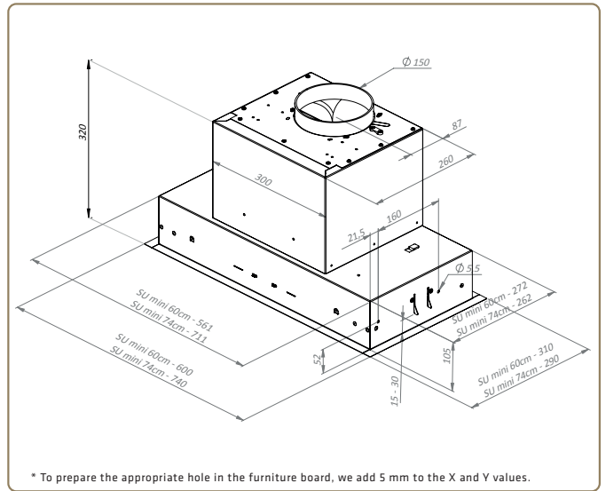
SU MINI - 60 cm / 74 cm
