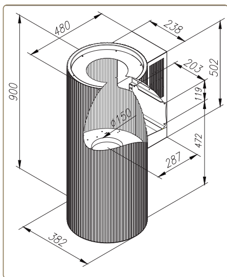
MONOGRAM
