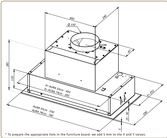
AURA - 55 cm / 74 cm
