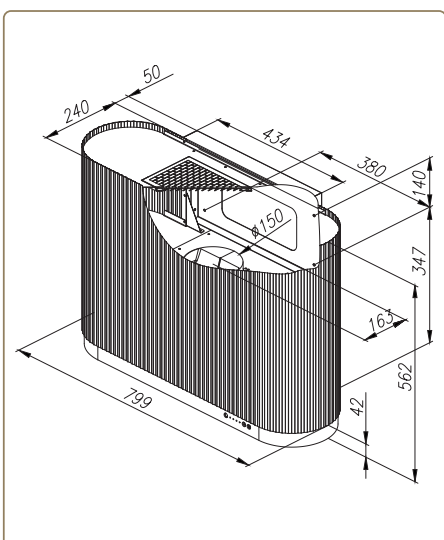
MONO - 80 cm
