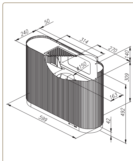
MONO - 60 cm
