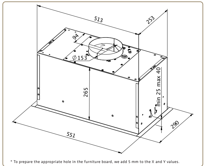
UNO - 55 cm
