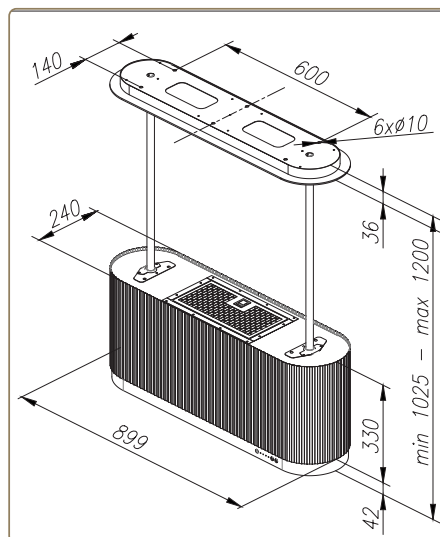
MONO W
