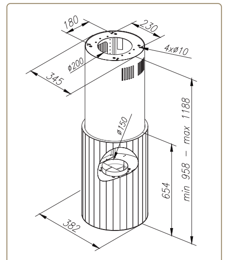
ROTO W
