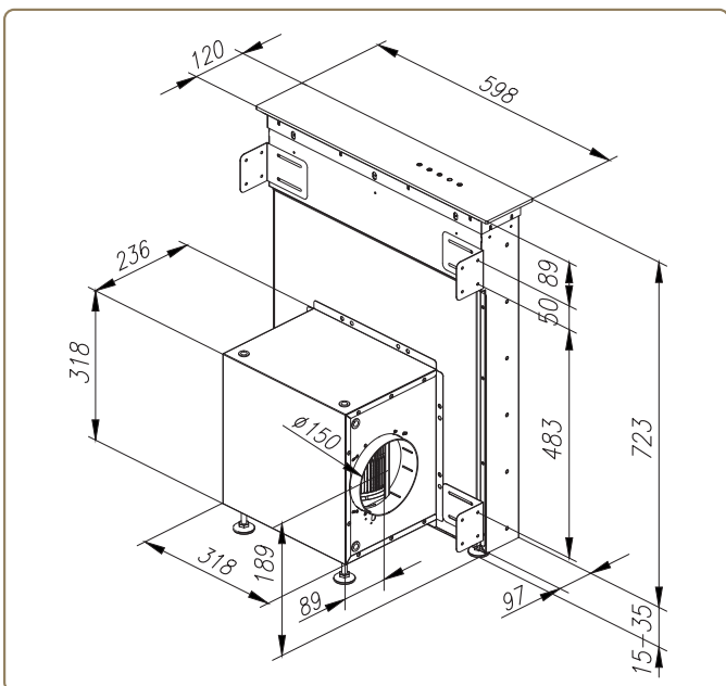
MOONDRAFT / 60 CM
