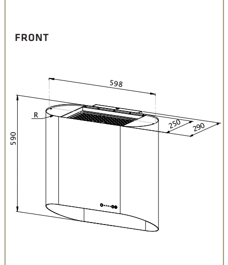
SIMPLE
