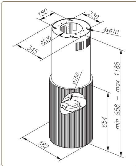
MONOGRAM W
