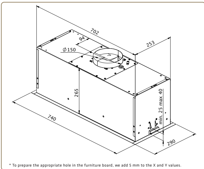
UNO - 74 cm
